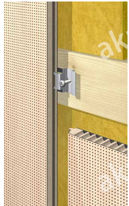
Detail vertikale Montage mit Montageclip
